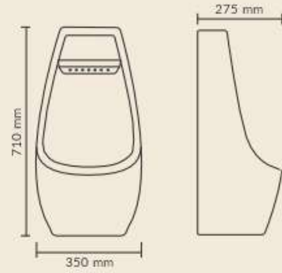
KENA Product : Urinal Dimensions : 350 X 275 X 710 mm
