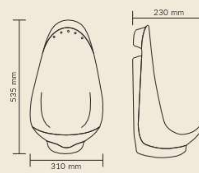
KENT Product : Urinal Dimensions : 310 X 230 X 535 mm
