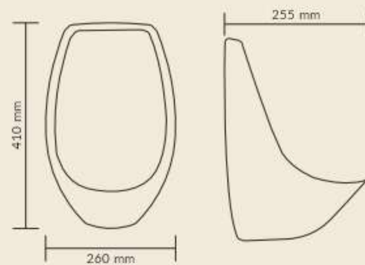
MINI LARGE Product : Urinal Dimensions : 260 X 255 X 410 mm
